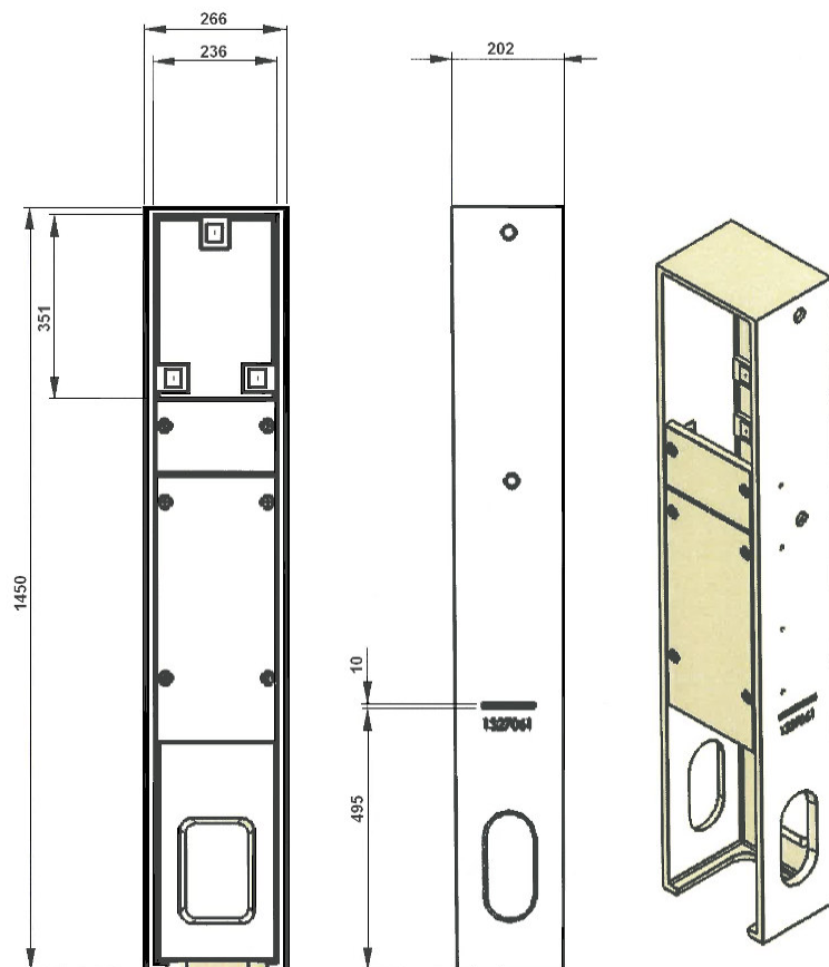
Coquille borne. Référence réséda : codet ENEDIS 13.27.048
