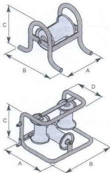
Galets prévus pour le déroulage du câble.
