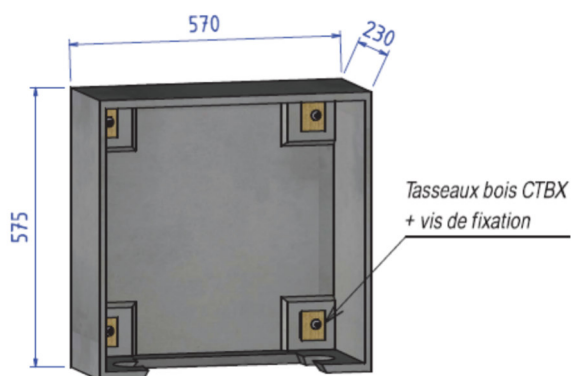
Coquille d'encastrement Référence réséda : codet ENEDIS 13.27.038
