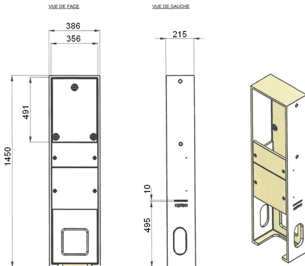
Coquille borne. Référence réséda : codet ENEDIS 13.27.048
