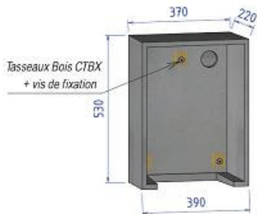
Coquille d'encastrement Référence réséda : codet ENEDIS 13.27.027
